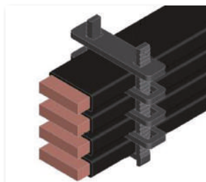
Ammarraggio universale con \Omega FLAT PER BARRE FLESSIBILI COFLEX, vedere pag. 54
