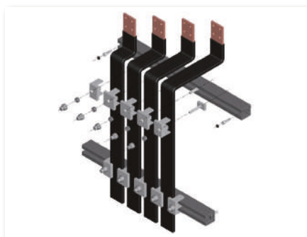
Ammarraggio universale con \Omega FLAT PER BARRE FLESSIBILI COFLEX, vedere pag. 54
